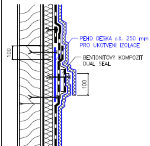
DETAIL "A" - II. ETAPA:
