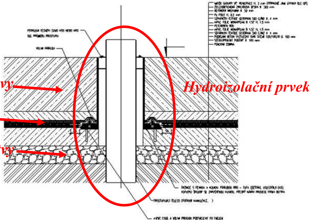
ŘEŠENÍ PROSTUPU POTRUBÍ VODOROVNOU HYDROIZOLACÍ M 1:5
